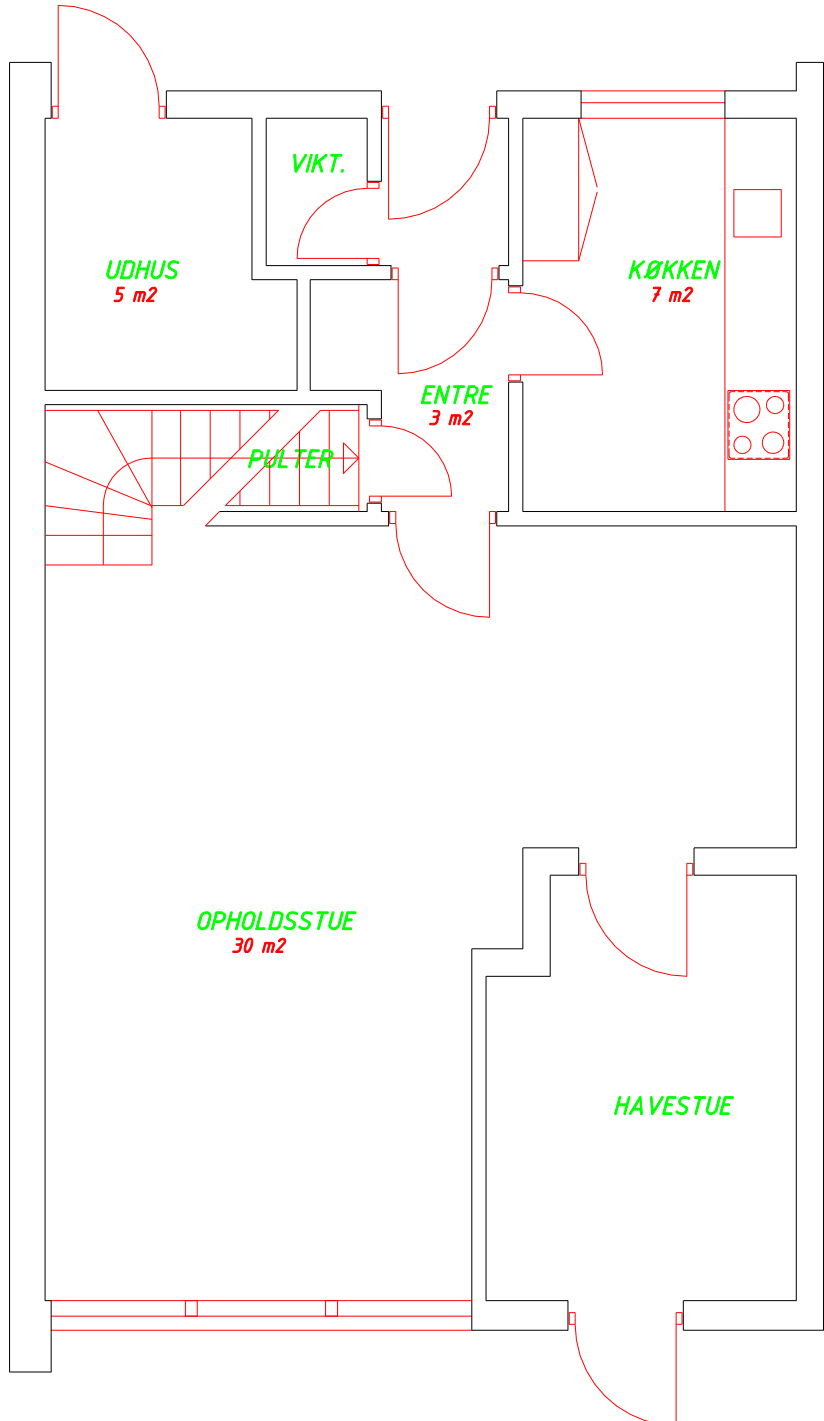
STUEPLAN
