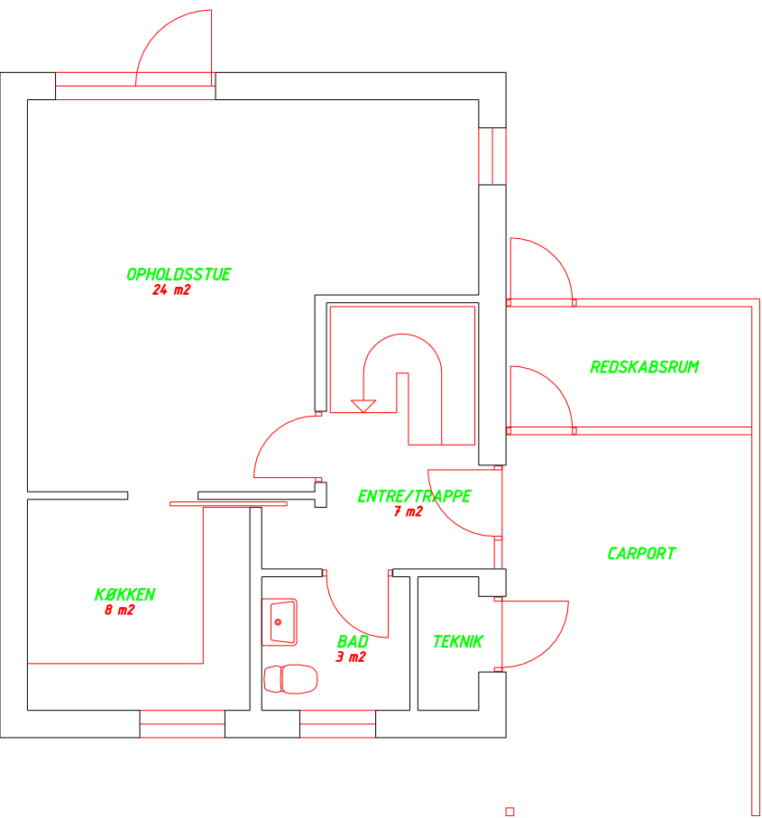
STUEPLAN — 4 VÆRELSE
