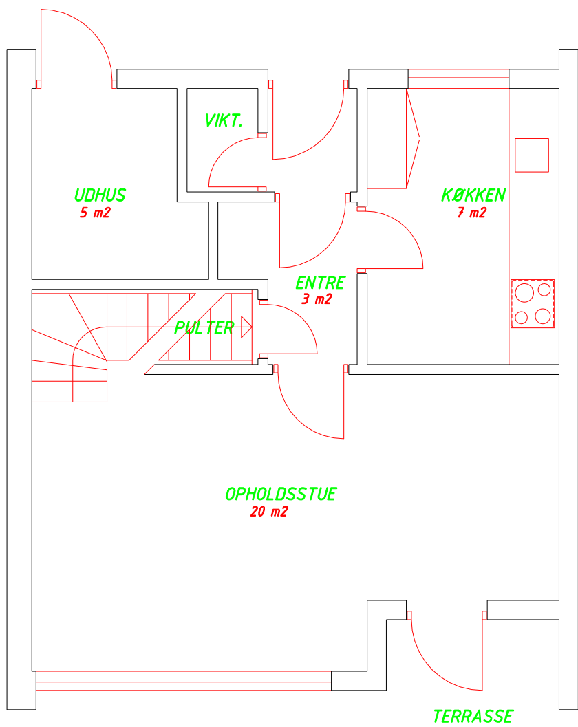
STUEPLAN
