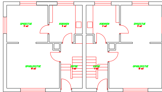
STUEPLAN — 4 VÆRELSE
