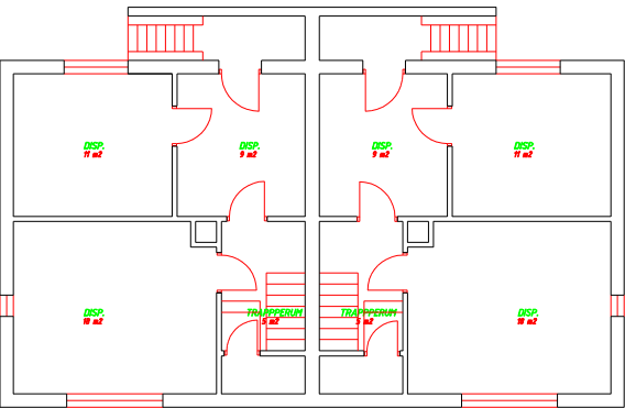
KÆLDERPLAN — 4 VÆRELSE
