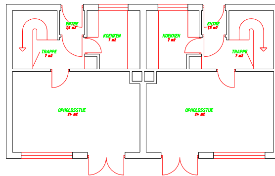
STUEPLAN – 3 VAERELSER
